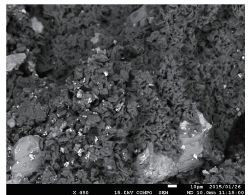
沖縄トラフの熱水活動域海底下から得られた堆積物試料中に見出された硫化鉱物。走査電子顕微鏡の反射電子組成像では、原子番号が大きい金属元素の鉱物が白っぽく見える。
